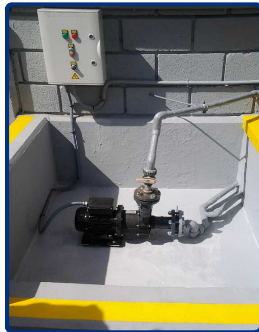
Montaje de Bomba Magnética y Cuadro de Suministro en cubeto independiente
