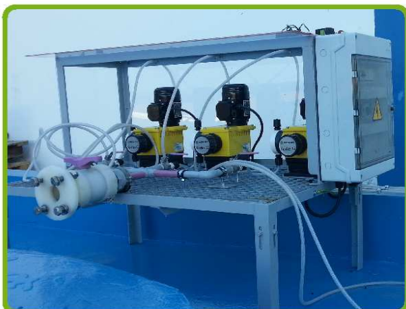
Detalle de Estructura Anti-salpicaduras para la Conexión de Suministro de tres bombas dosificadoras en PVC tratado con fibra de vidrio y esmalte
